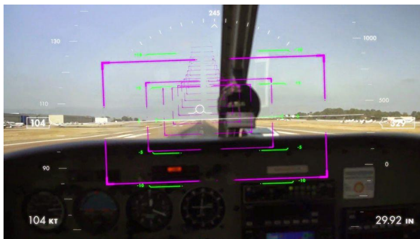
Abbildung 51: Beispielhafte Informationseinblendung per HMD (Aeroglass / Screenshot Imagevideo [186])
